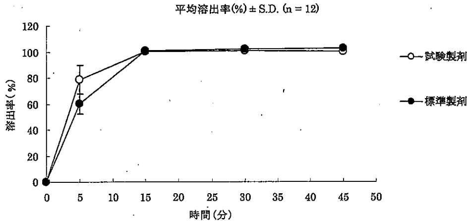
図*** 試験剤及び標準剤の平均溶出曲線
