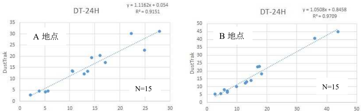
図 2 2018 年 1～2 月の試験結果 (24 時間平均 単位: \mu\text{g}/\text{m}^3 ) (横軸は自動測定機による濃度, 縦軸は DustTrak)
