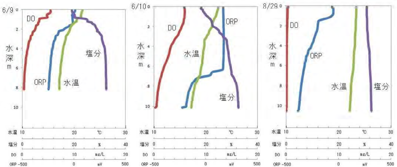
図 2 6/9, 6/10の船橋港の水質鉛直プロファイル
