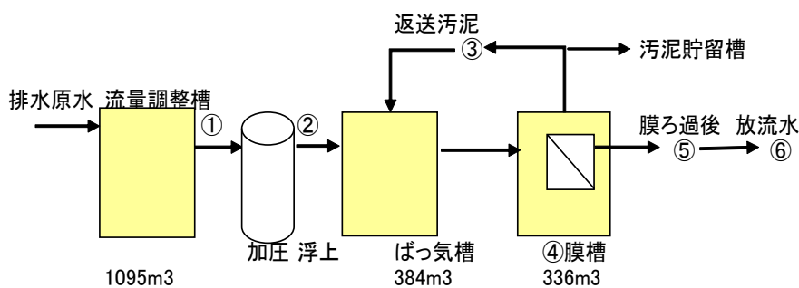
図1 排水処理工程
