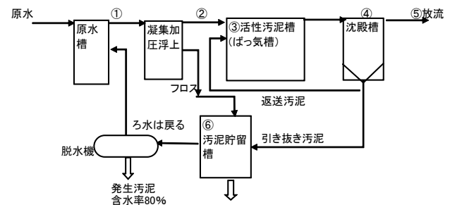
図1 処理工程図
