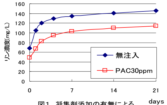
図1 凝集剤添加の有無によるリン濃度変化
