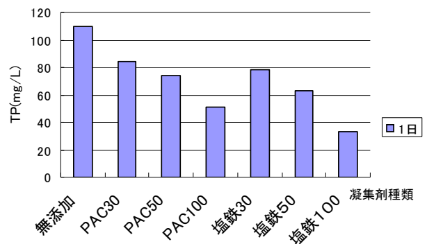
図3 凝集剤量と汚泥のろ液中りん濃度[1日後]
