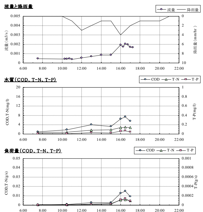
図2 流量・水質調査結果 (⑨山林：天辺地区)
