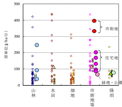
図3 COD原単位
