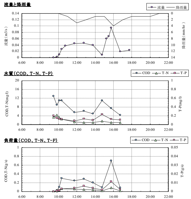
図1 流量・水質調査結果 (③住宅地：佐倉白銀ニュータウン)
