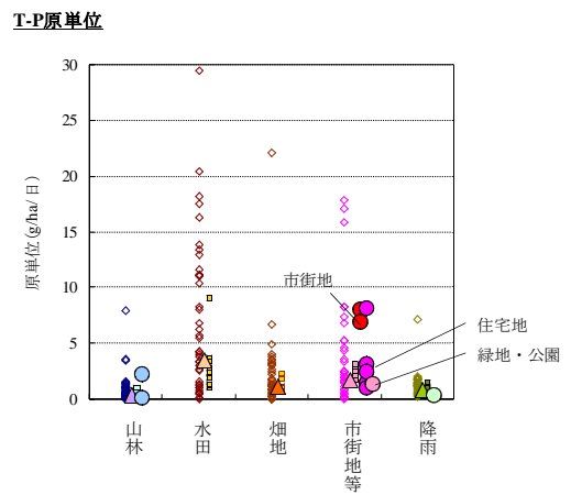
図5 T-P原単位
