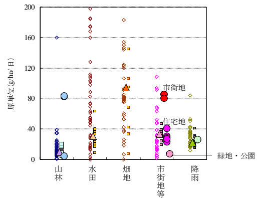
図4 T-N原単位
