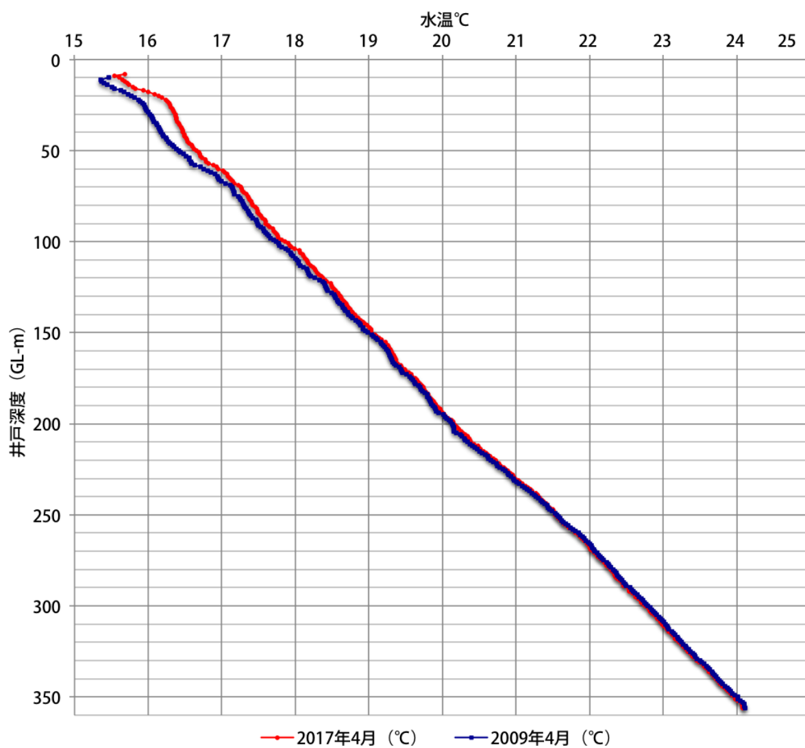
図 WTG-1 観測井（柏市箕輪新田 井戸深度：356m）における孔内地下水温度分布
