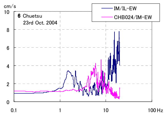
図2 主要動における周波数スペクトル
