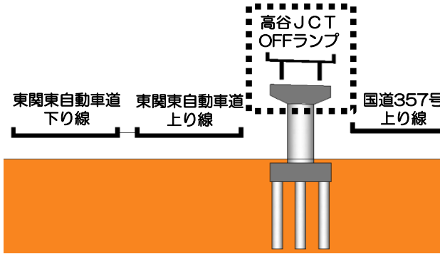
工事範囲（高谷ジャンクション橋南）
