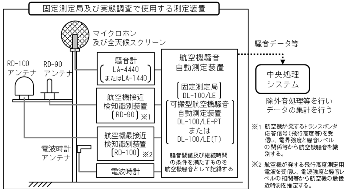
図2 基本構成図
