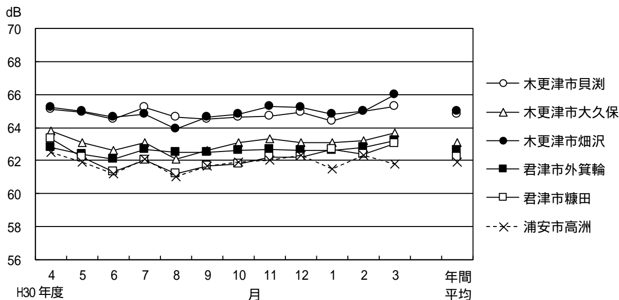
図3 最大騒音レベルの月間のパワー平均値
