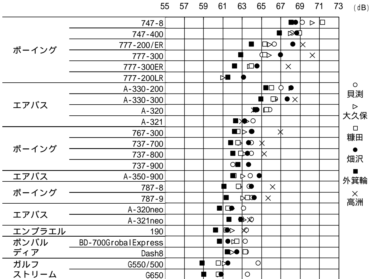
図6 機種別最大騒音レベルのパワー平均値
