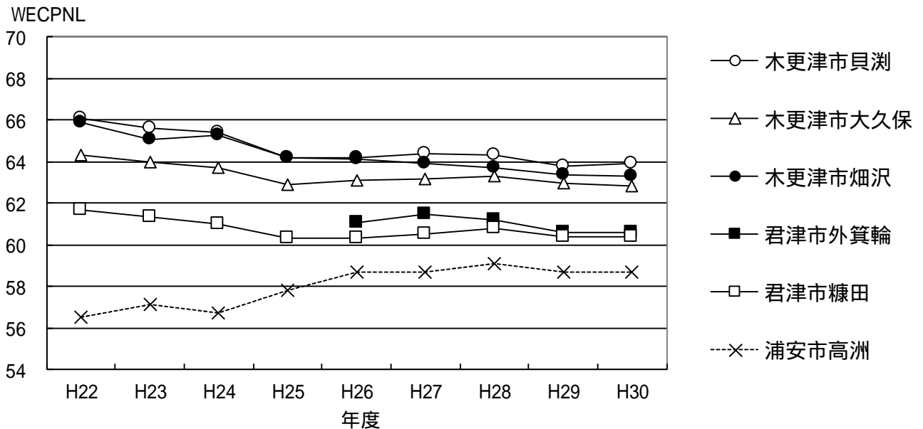
図10 WECPNLの経年変化
