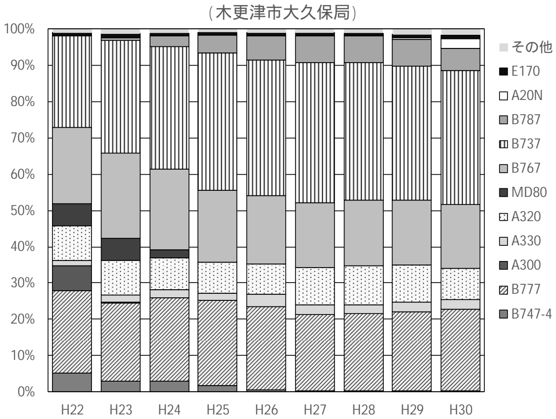
図 11 騒音発生回数の機種区分別割合の経年変化
