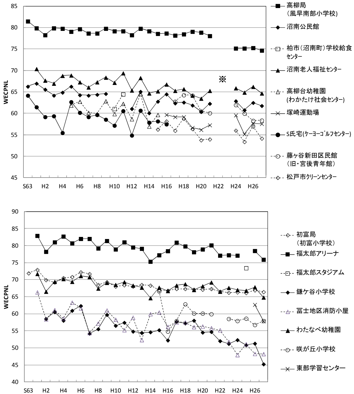
図5 年間 WECPNL の経年変化（上段：飛行場北側、下段：飛行場南側）
