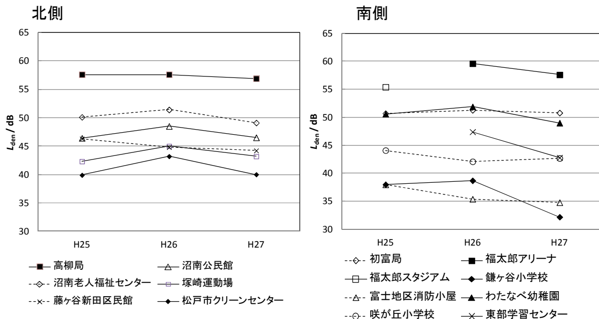
図4 年間 L_{den} 推計値の経年変化
