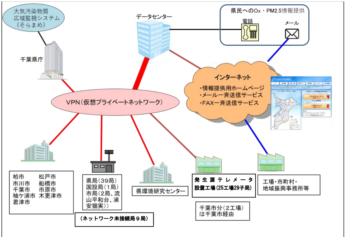
千葉県大気情報管理システム ネットワーク構成図(2022年4月1日現在)
