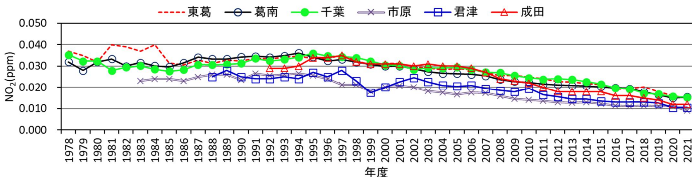
図2-2-8 NO 2 年平均値の推移(自排局)
