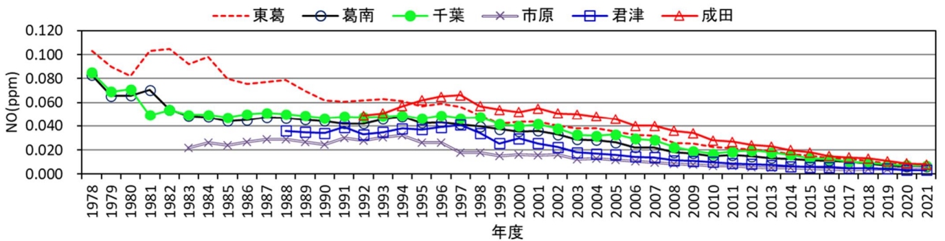
図2-3-8 NO年平均値の推移(自排局)
