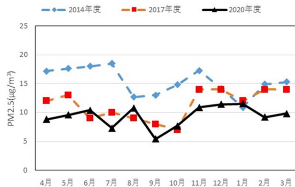
図2-7-4 PM2.5月平均値の経月変化(自排局)
