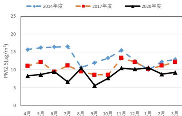
図2-7-3 PM2.5月平均値の経月変化(一般局)
