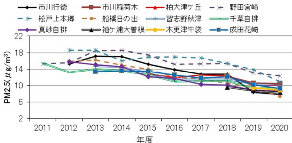
図2-7-6 PM2.5年平均値の推移(自排局) 局名の(車)は省略
