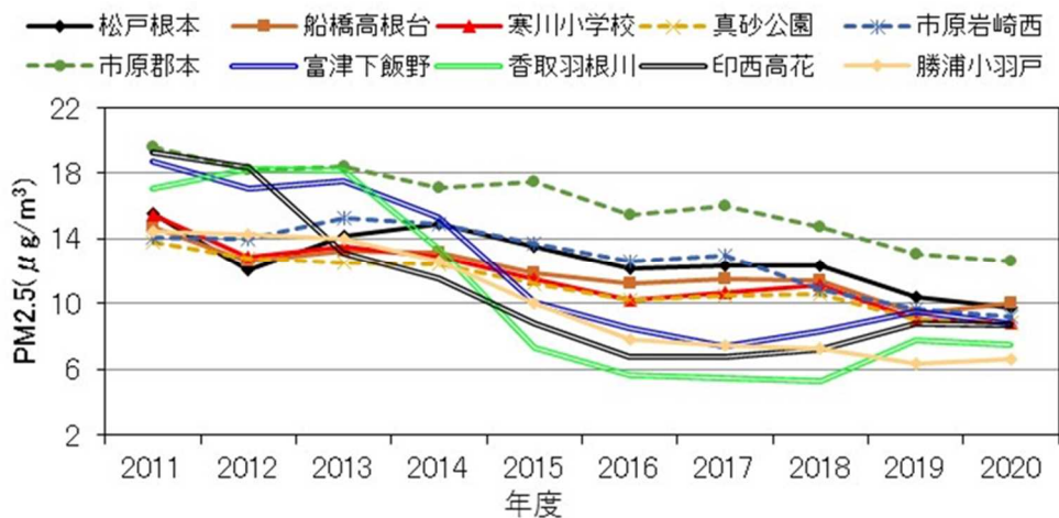
図2-7-5 PM2.5年平均値の推移(一般局)
