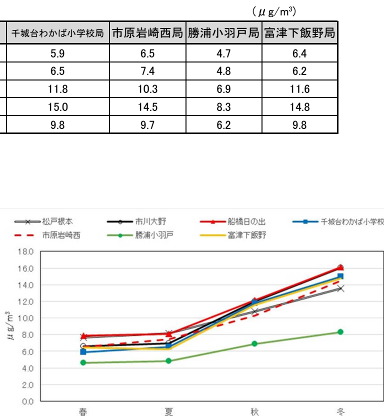
図 2-7-8 PM2.5質量濃度の季節変化
