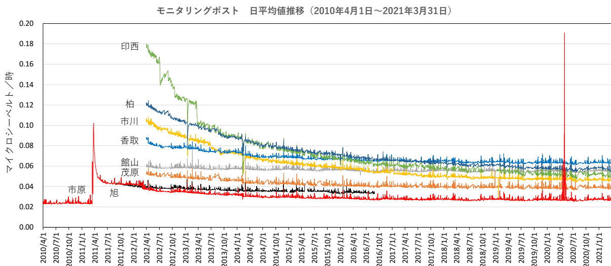
図5-2 空間線量率の推移(日平均値)
