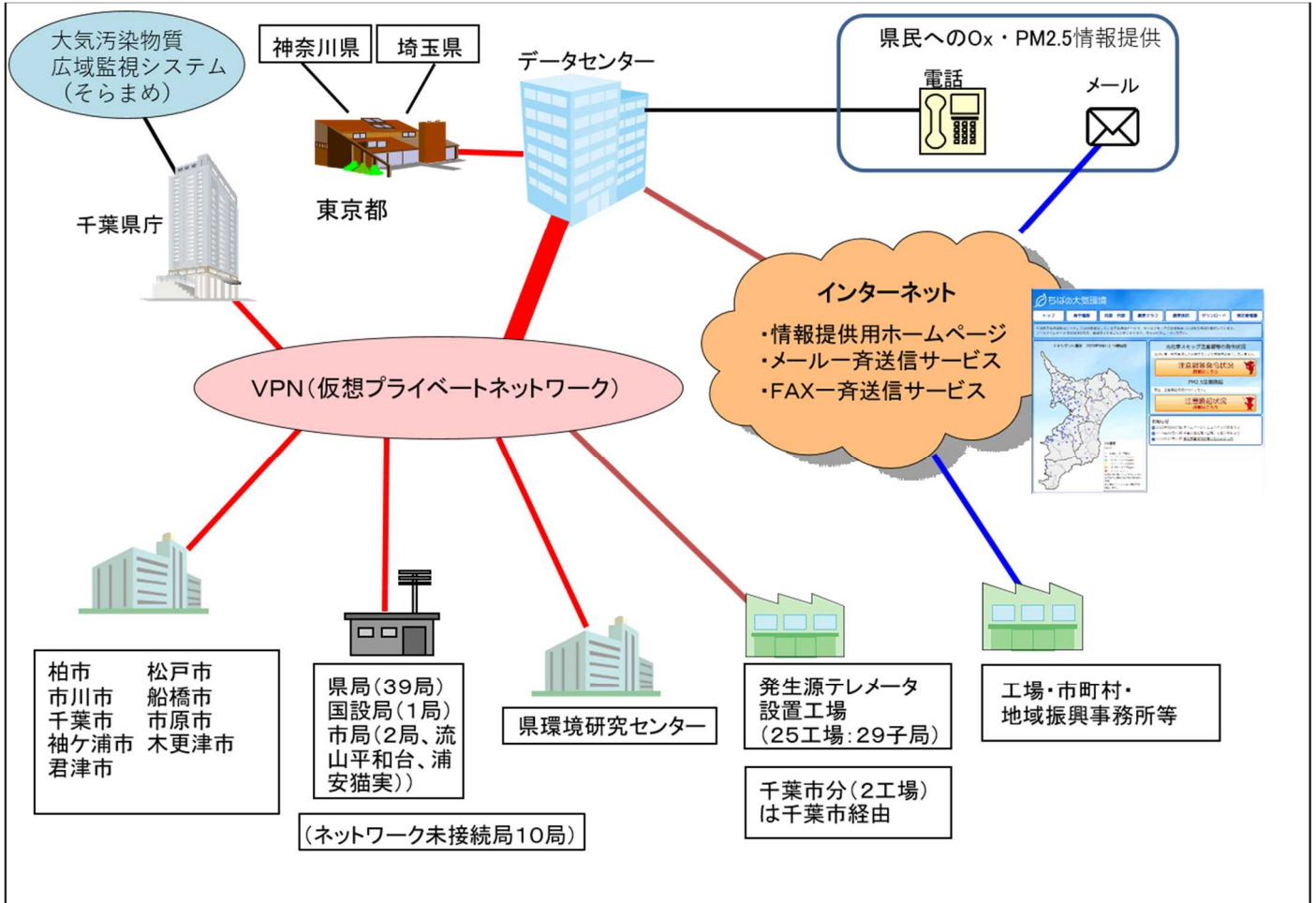
千葉県大気情報管理システム ネットワーク構成図(2019年4月1日現在)
