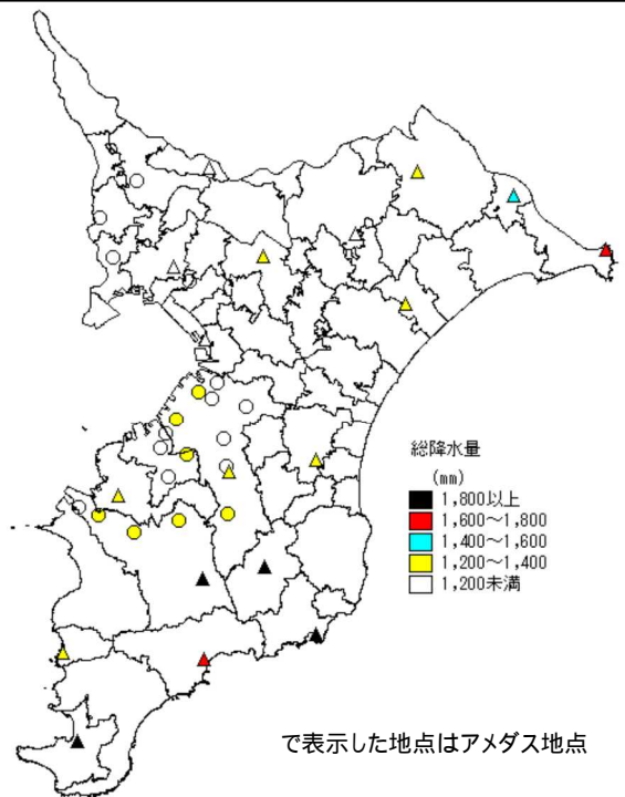
図1-4-2 降水量の分布(アメダス含む)
