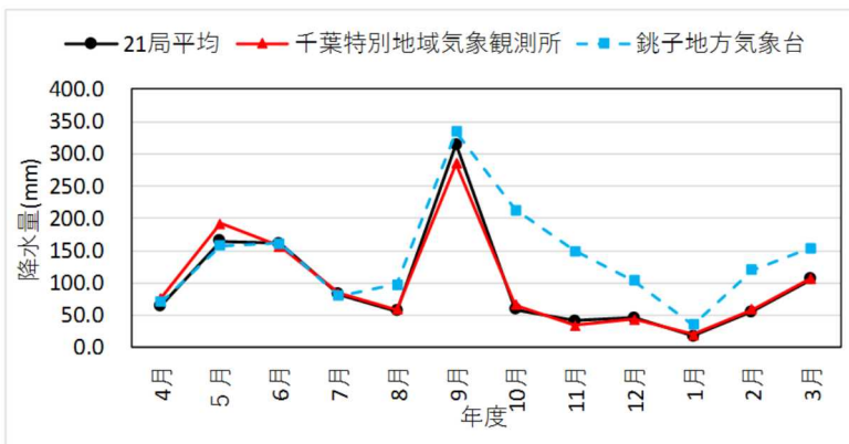
図1-4-1 月降水量の経月変化(県内21局平均)
