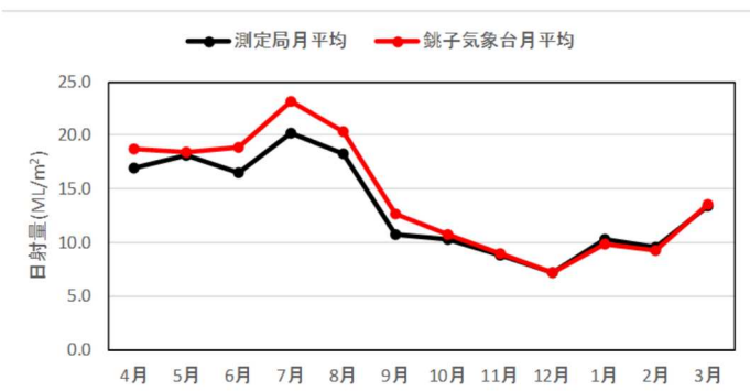
図1-2-1 日合計月平均値の経月変化
