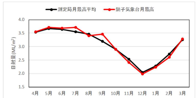
図1-2-2 月最高値の経月変化
