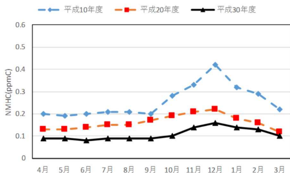
図2-8-6 NMHC月平均値の経月変化(一般局)
