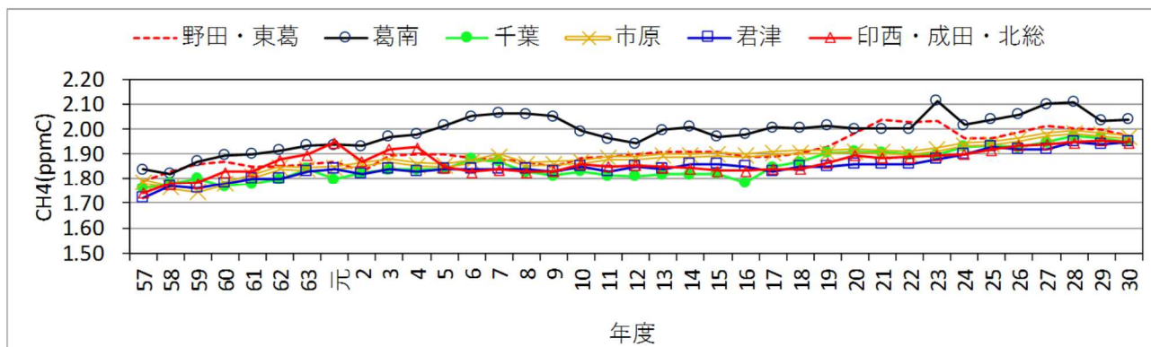
図2-8-9 CH 4 年平均値の推移(一般局)
