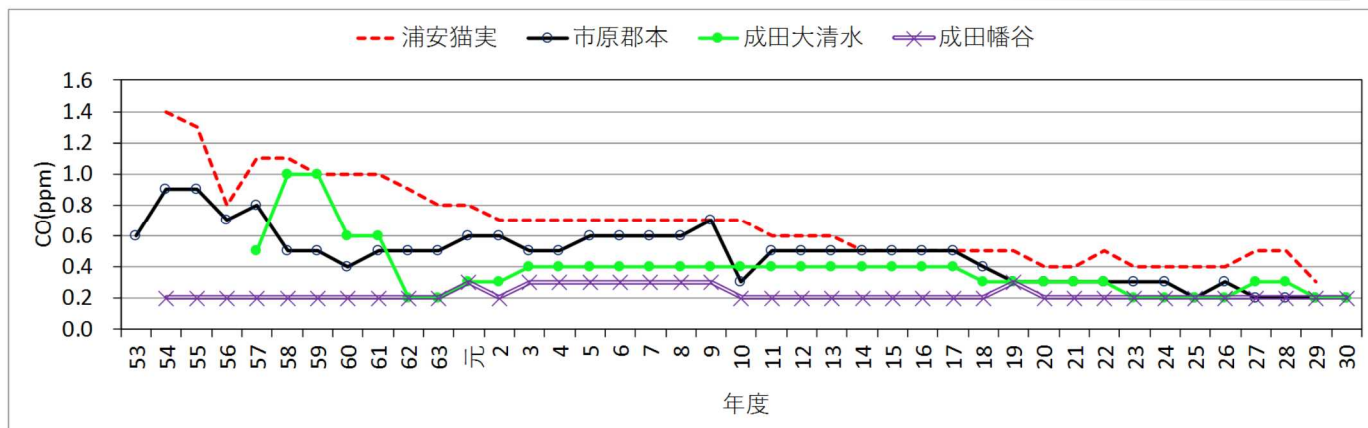
図2-4-5 CO年平均値の推移(一般局) 昭和53年度から平成30年度の間に25年以上測定している4局の年平均値。
