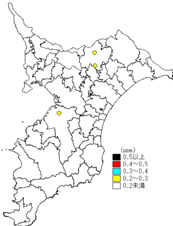
図2-4-1 CO年平均値の分布(一般局)
