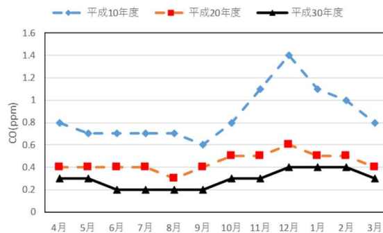
図2-4-4 CO月平均値の経月変化(自排局)
