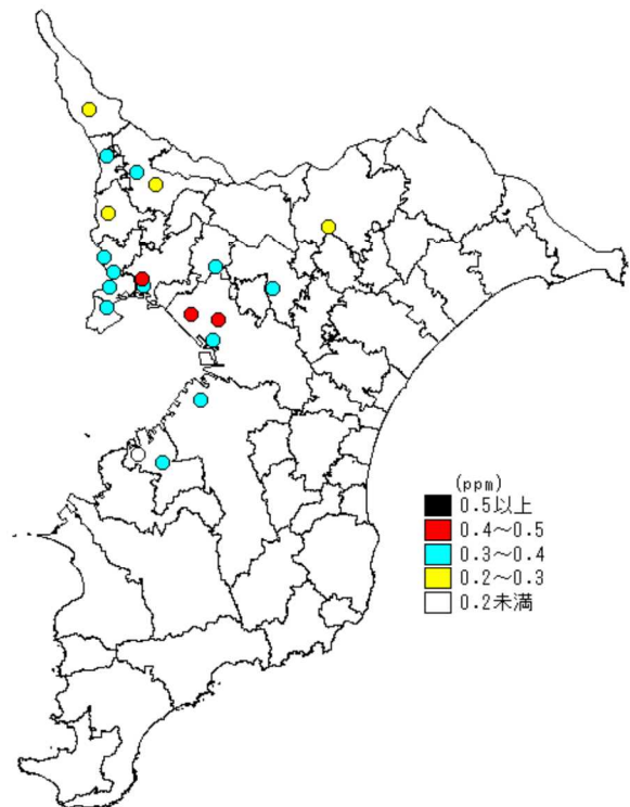
図2-4-2 CO年平均値の分布(自排局)
