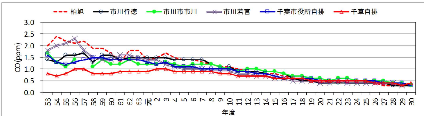
図2-4-6 CO年平均値の推移(自排局) 昭和53年度から平成30年度の間に25年以上測定している6測定局の年平均値。局名の(車)は省略。
