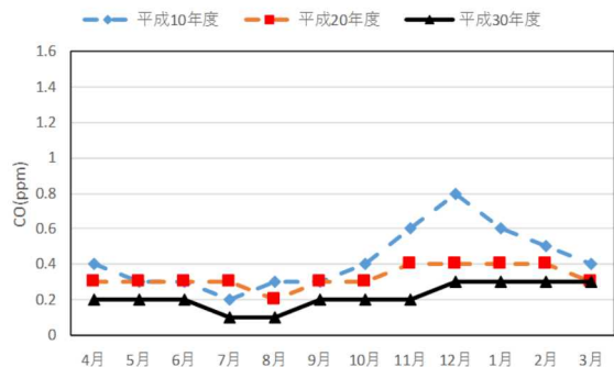
図2-4-3 CO月平均値の経月変化(一般局)
