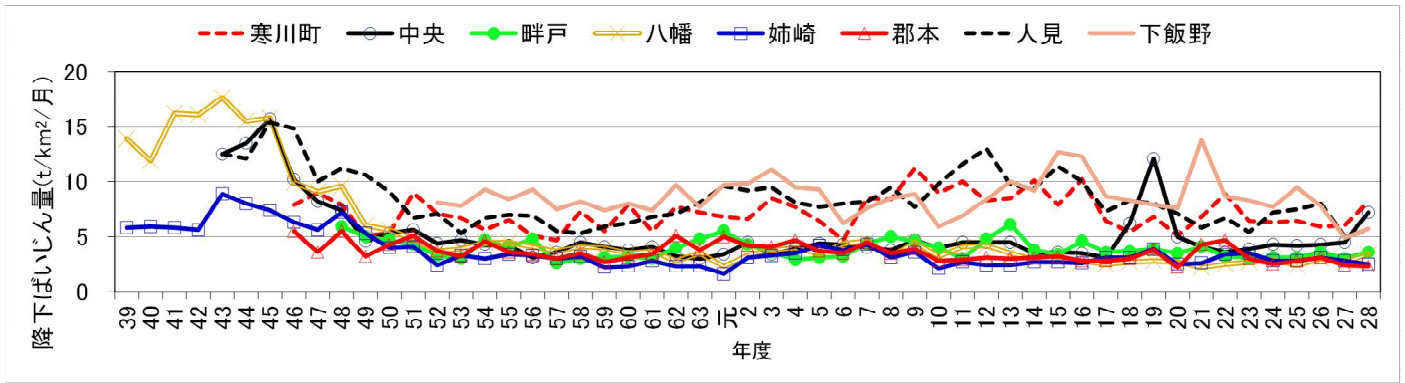
図3-3 ばいじん量年平均値の推移
