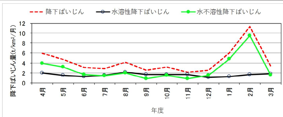
図3-2 総ばいじん量、水溶性降下ばいじん量、水不溶性降下ばいじん量の経月変化
