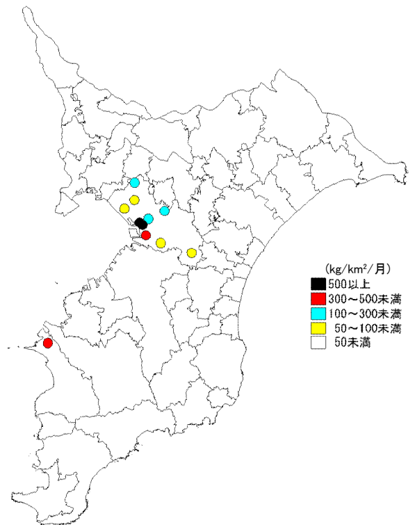
図3-9 Fe量の分布
