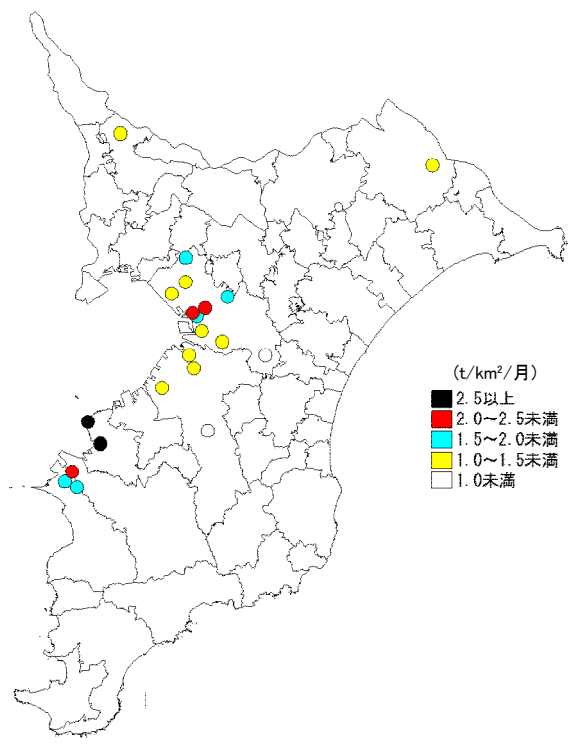
図3-5 水溶性降下ばいじん量の分布
