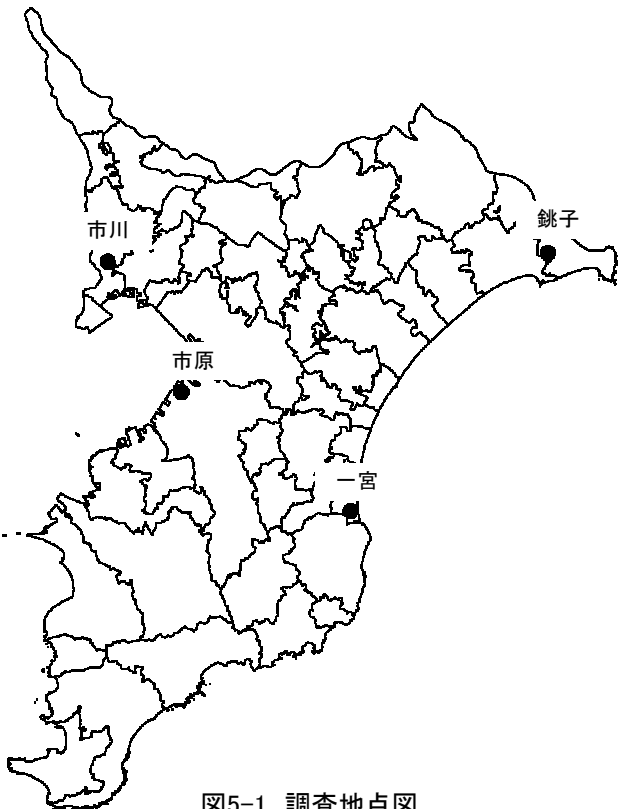
図5-1 調査地点図
