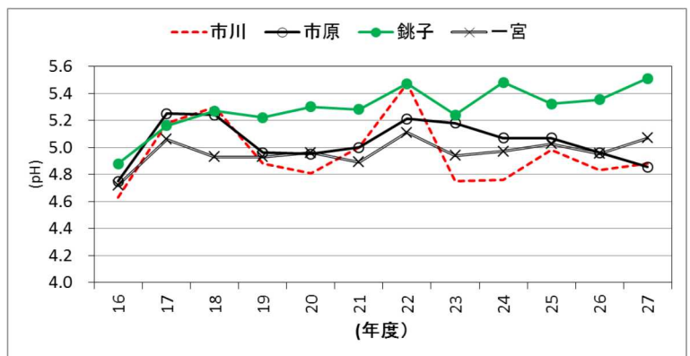
図5-2 pHの経年推移
