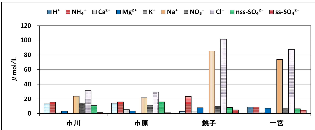
図5-3 降水中イオン成分の濃度
