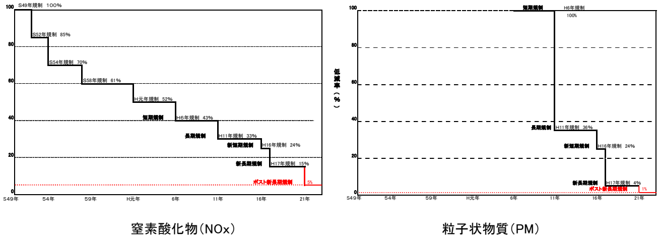
図1 自動車排出ガス規制の経緯(ディーゼル重量車)
