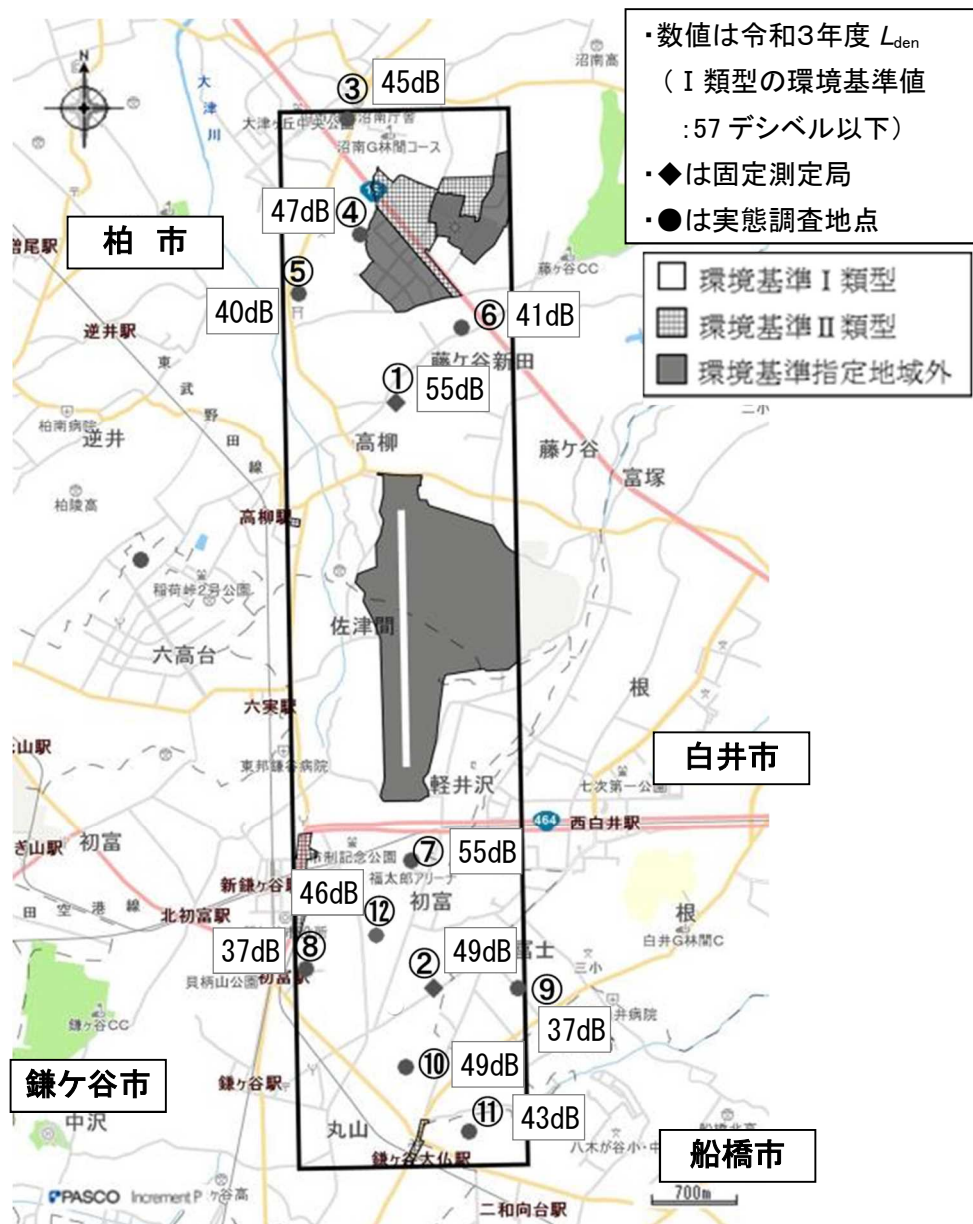
別図3 下総飛行場周辺における航空機騒音の固定測定局及び実態調査地点
