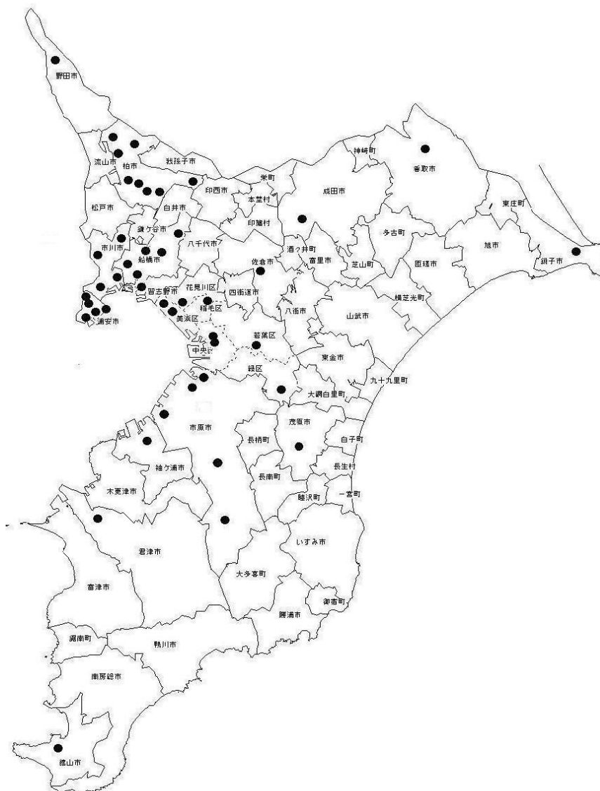
図1 大気中アスベスト濃度測定地点図（市町村区域は測定時期でのもの）
