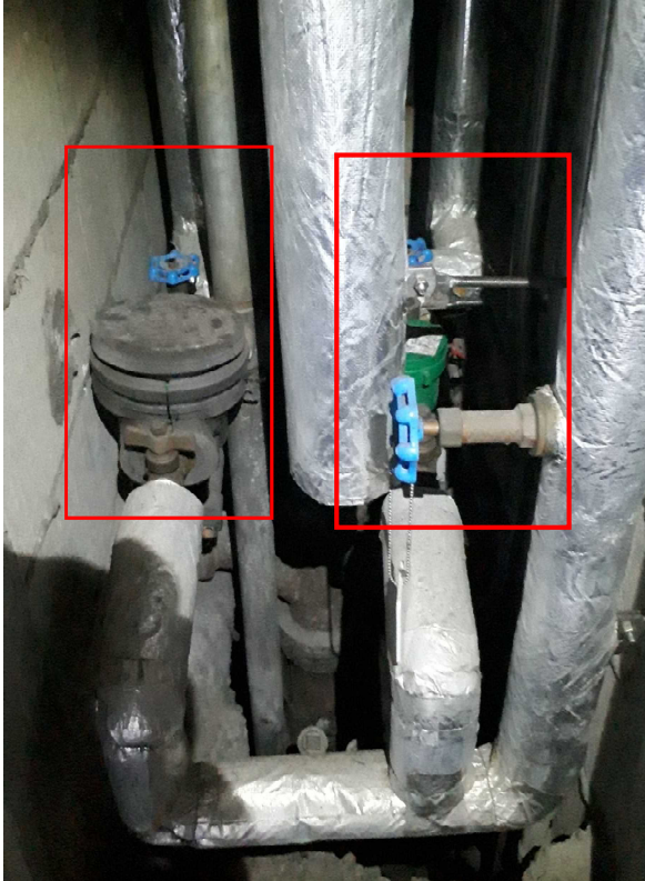
空気弁とバルブ 盗取前
