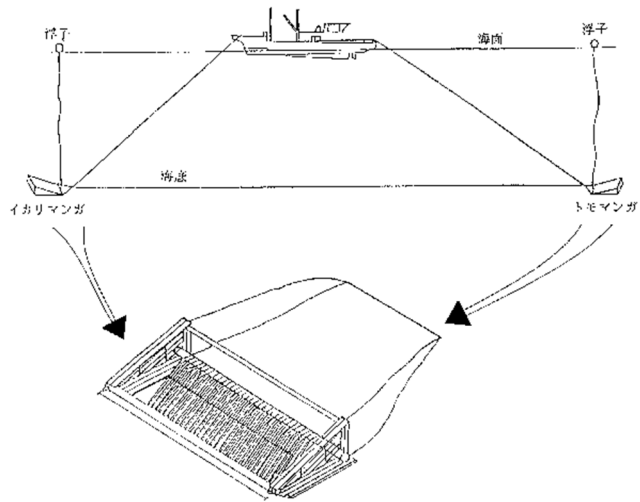
図3 貝桁網漁業
