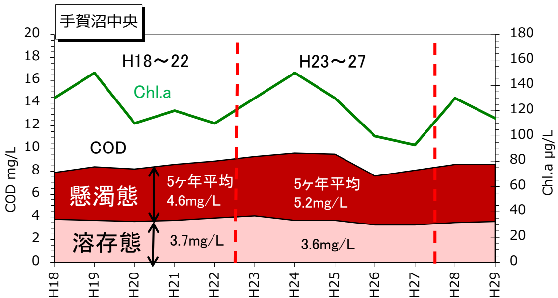
図2 手賀沼における各態CODの変化(年平均値)
