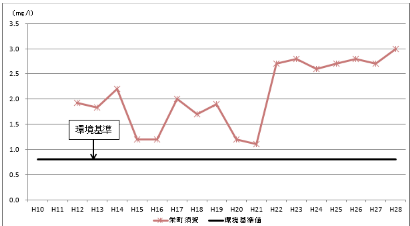
図 2 - 3 概況調査（定点観測）実施地点のふっ素濃度経年変化 （過去に環境基準超過のあった地点の抜粋）
