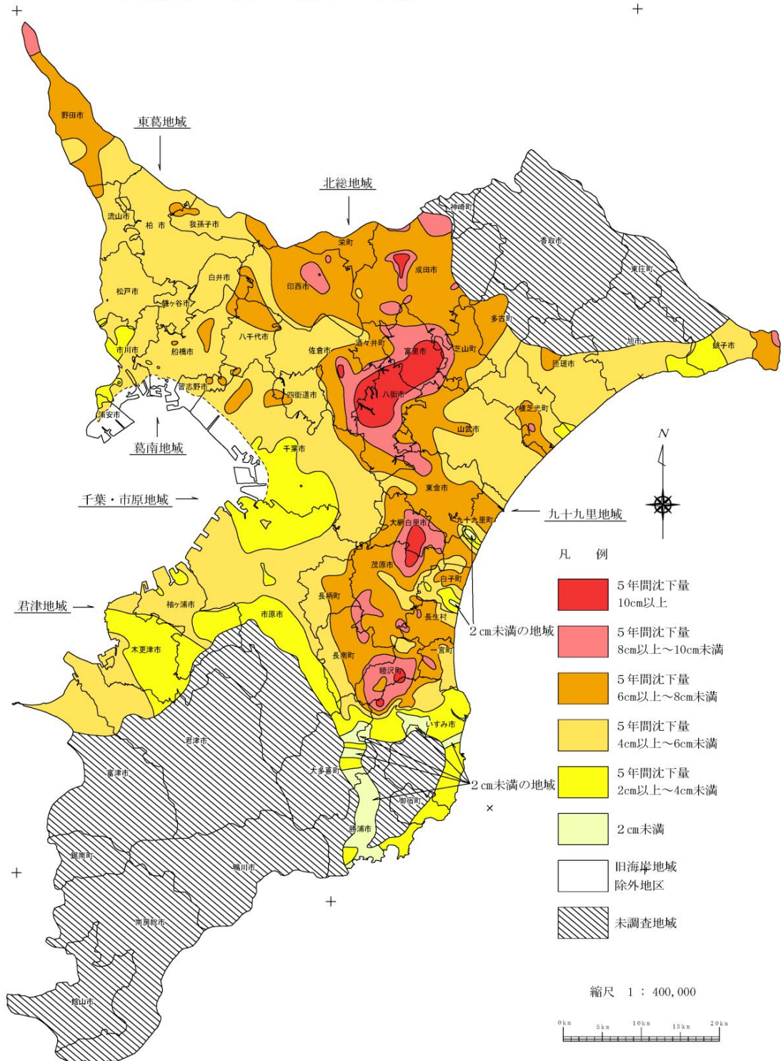
千葉県水準基標変動図 (5年間変動図) (平成22年1月～平成27年1月)
