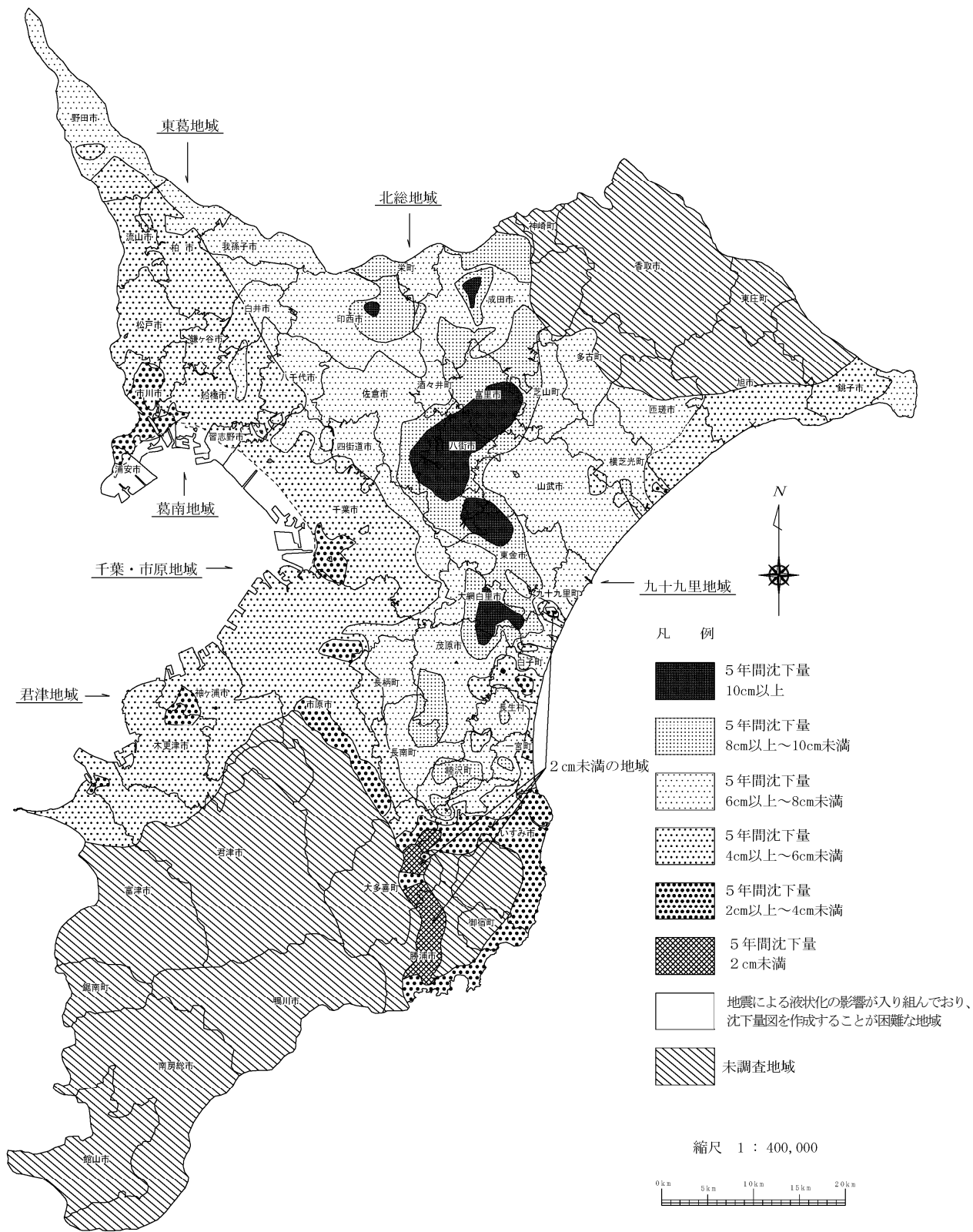
千葉県水準基標変動図 (5年間変動図) (平成20年1月～平成25年1月)
