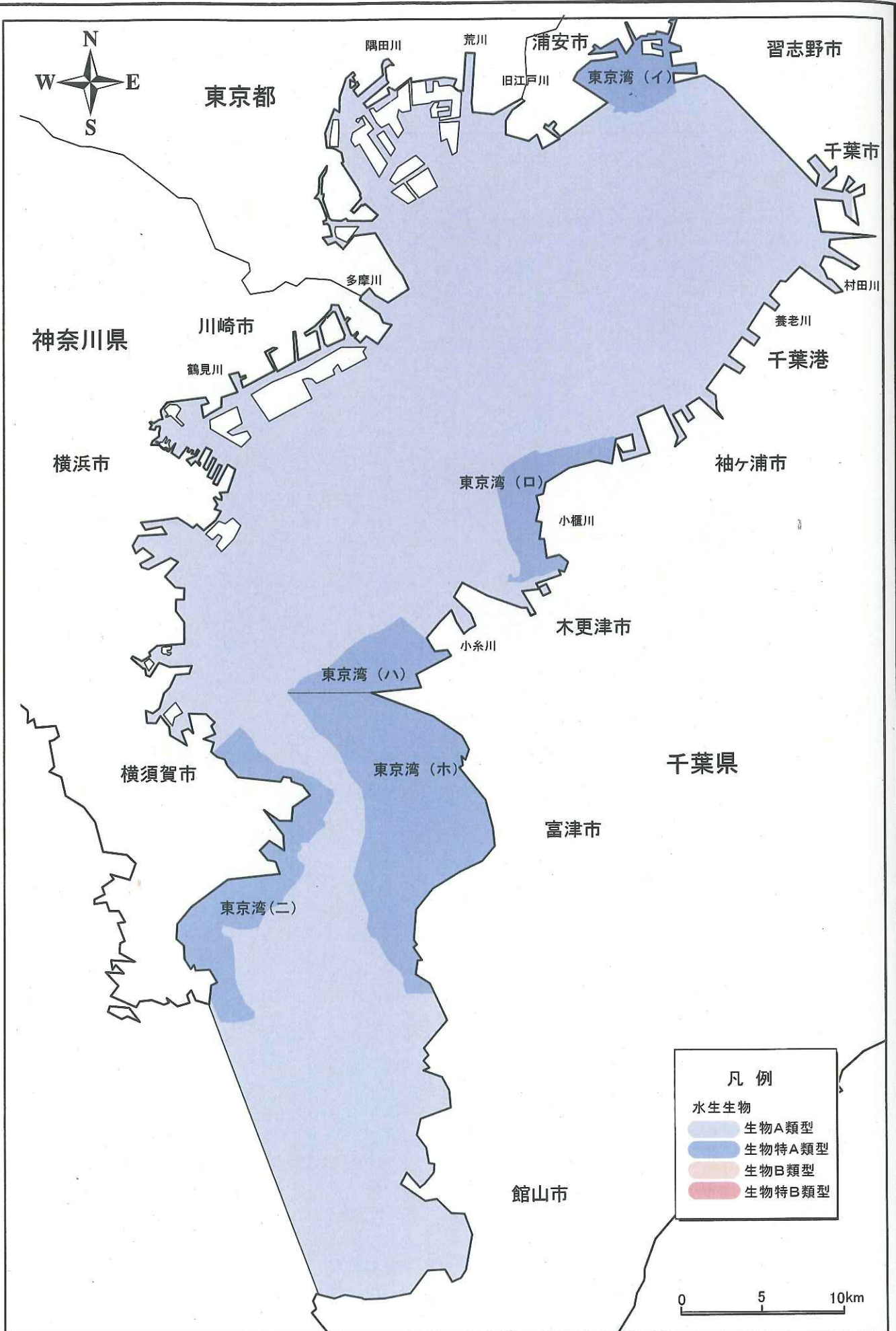
〔東京湾〕水生生物保全に関する海域類型指定概況図
