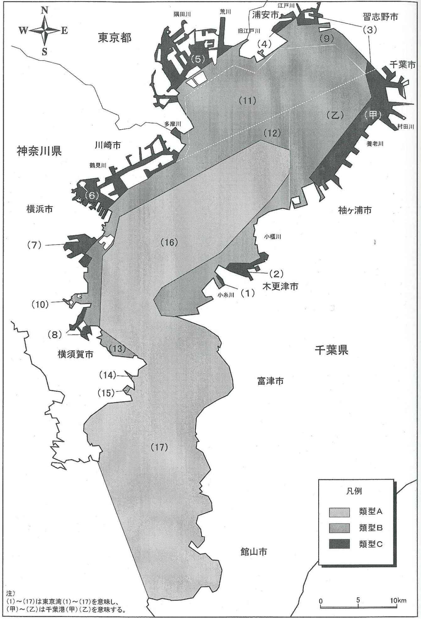
〔東京湾〕 COD等に関する海域類型指定概況図
