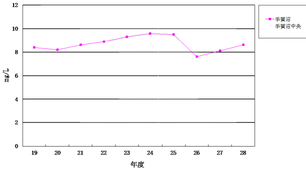
図1-10 手賀沼水質（COD年平均値）経年変化
