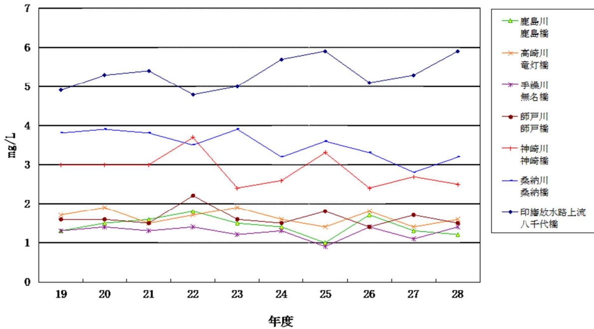
図1-9 印旛沼流入河川（環境基準点）水質（BOD年平均値）経年変化
