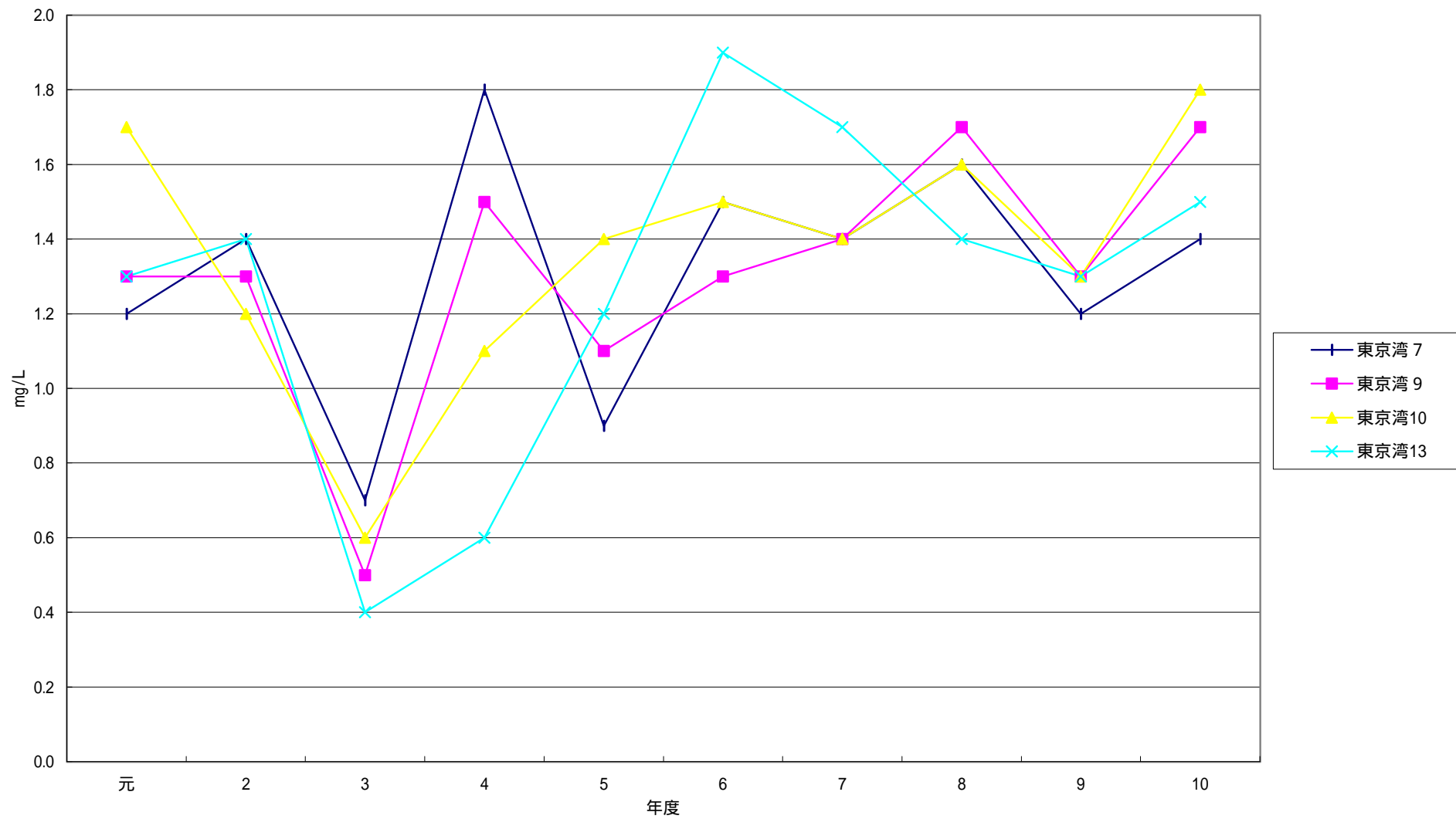
図 1 - 2 7 不溶解性COD推移
