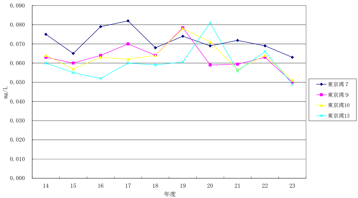
図1-27 全りん推移
