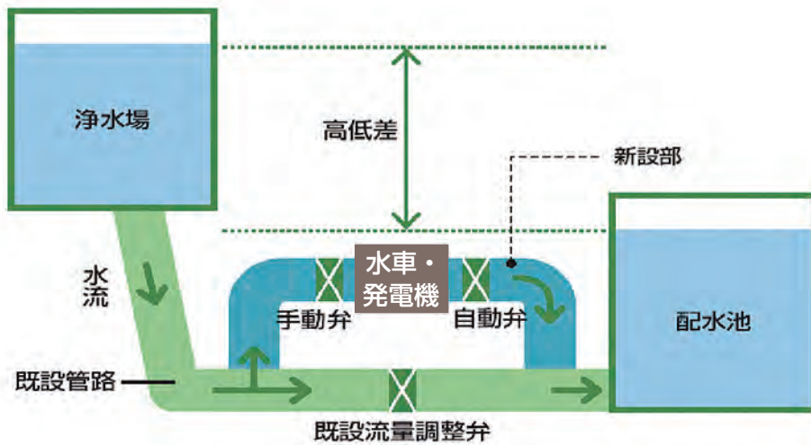
北船橋給水場の1号機マイクロ水力発電装置
