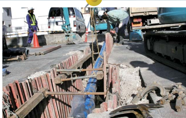
管路の工事 計画的な管路の更新・整備により、耐震化を進めています。
