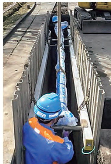
図V—7 配水管の布設替えの様子
