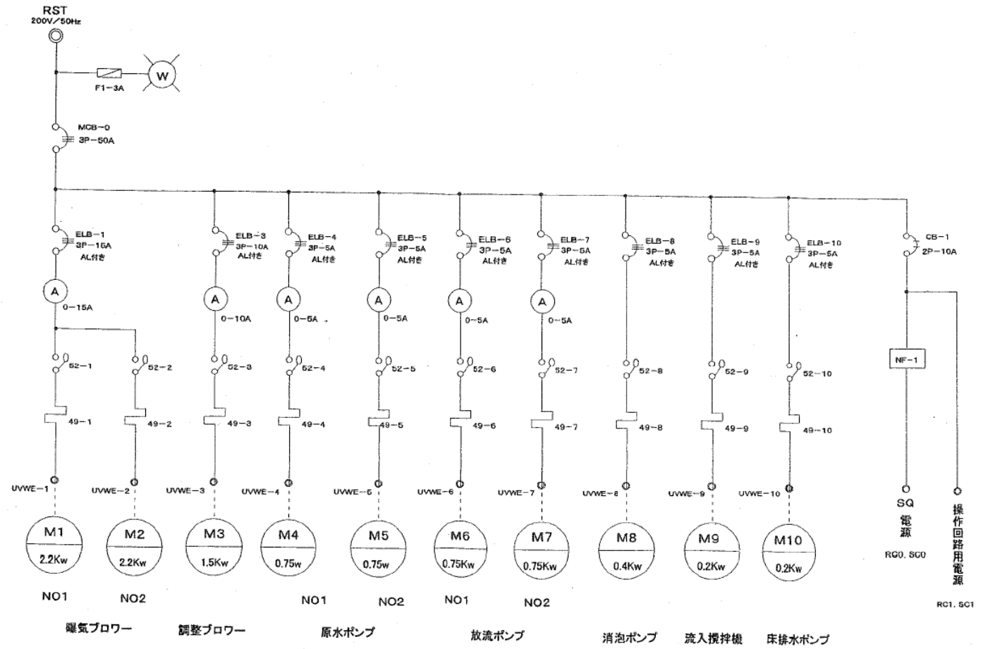
参考図 2-2 浄化設備動力回路図(現状)
