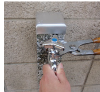
⑦ ハンドルをよくしめてから、スパナ等で上部をしっかりとしめつけます。これで完了です。止水栓を左↶に回して開けてください。
