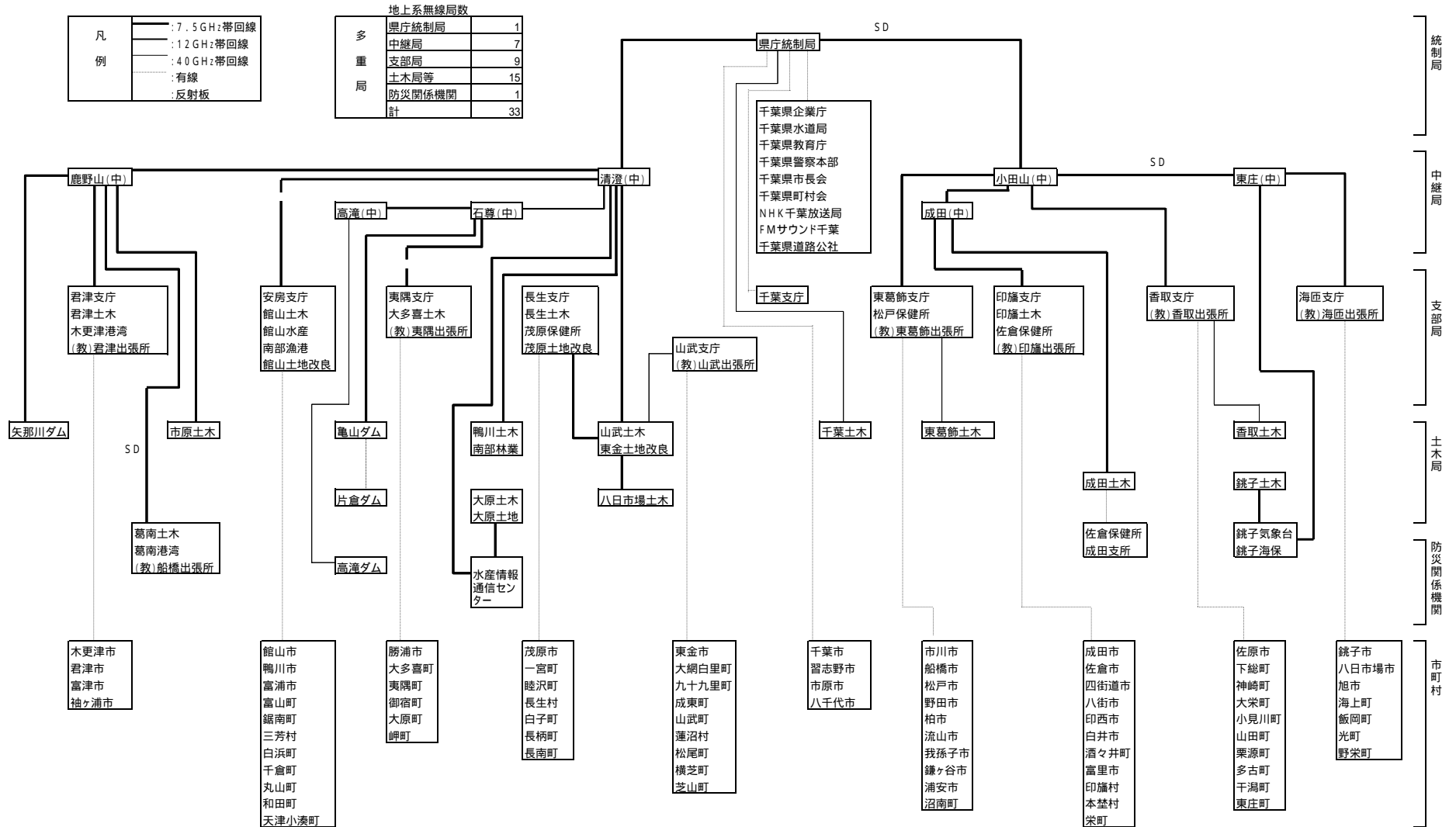
図1 防災行政無線地上系回線構成図(平成15年4月現在)
