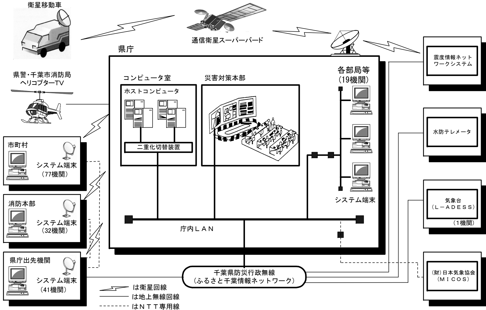
千葉県総合防災情報システム構成図
