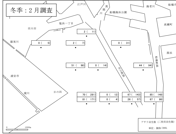
図 3.4.2 アサリおよび二枚貝浮遊幼生の分布状況
