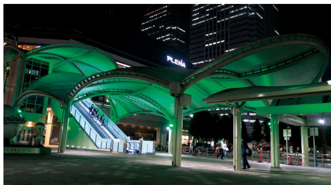
海浜幕張駅駅前広場シェルター
