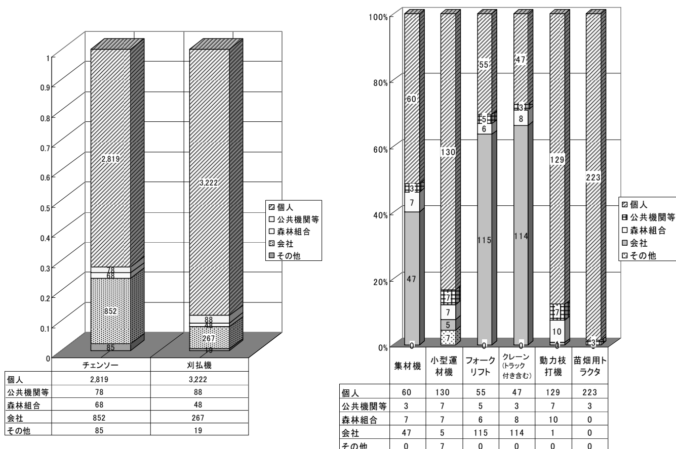
主な林業機械の保有状況（平成17年度）
