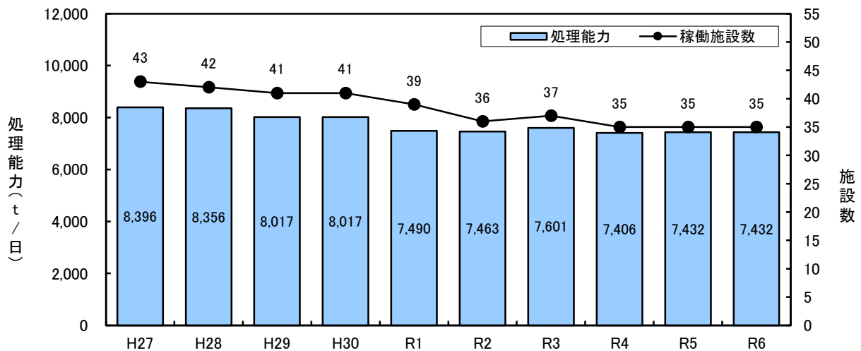
図-7 焼却処理施設の稼働施設数と処理能力の推移
