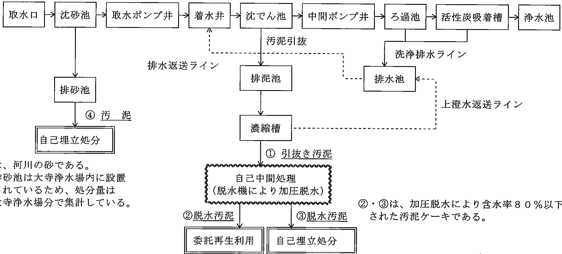
浄水処理工程図（十日市場浄水場）
